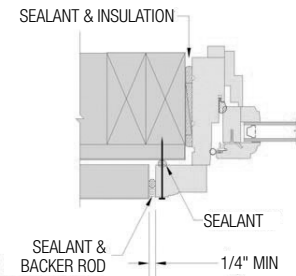
FIG. 19: SIDE JAMB
