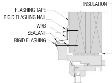
FIG. 15: HEAD JAMB
