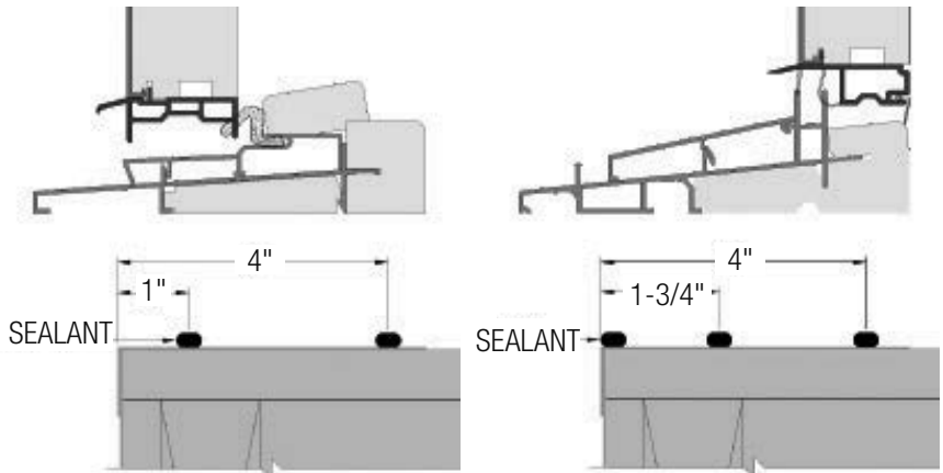
FIG. 9: OUT-SWING PATIO DOOR SILL
