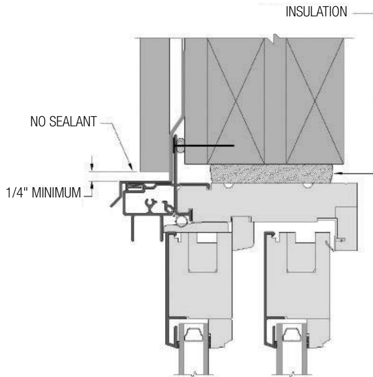
FIG. 25: SLIDING HEAD JAMB
