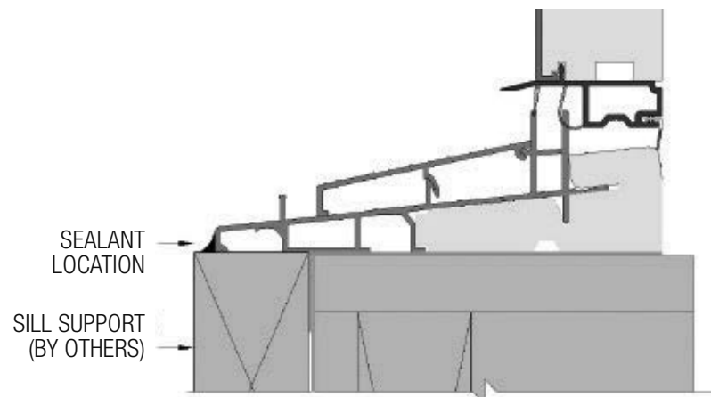
FIG. 16: STANDARD DOOR SILL
