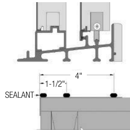
FIG. 11: SLIDING PATIO DOOR SILL
