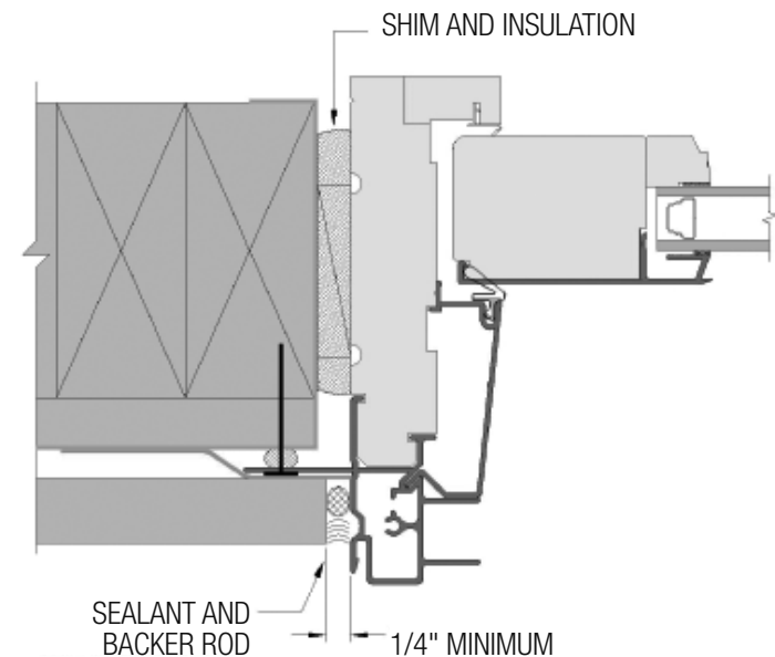
FIG. 24: SIDE JAMB
