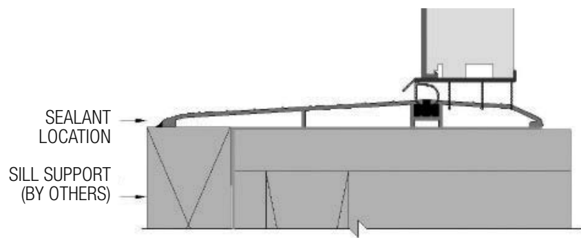
FIG. 17: HANDICAP DOOR SILL
