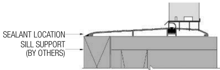
FIG. 16: HANDICAP DOOR SILL
