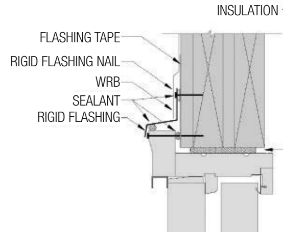
FIG. 18: HEAD JAMB
