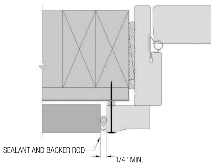
FIG. 20: SIDE JAMB
