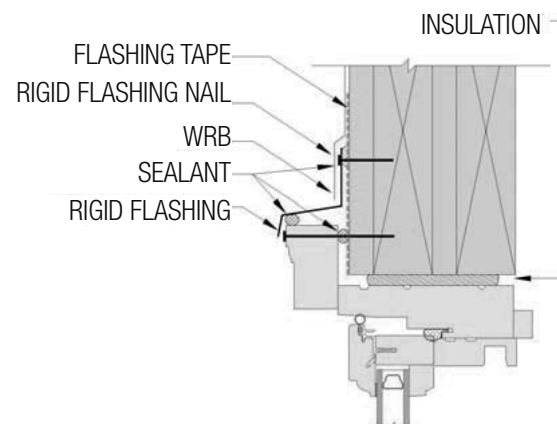
FIG. 15: HEAD JAMB
