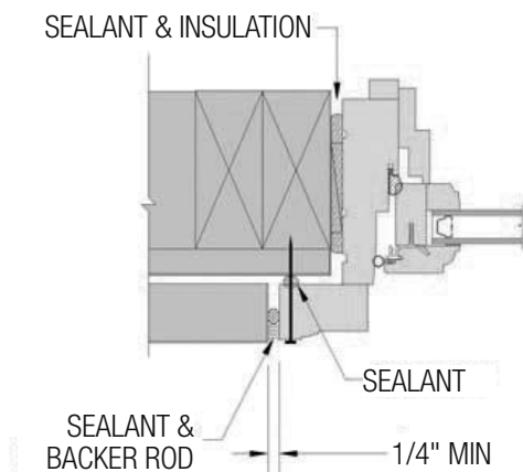
FIG. 19: SIDE JAMB
