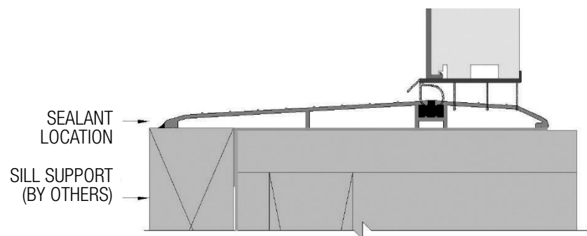
FIG. 17: HANDICAP DOOR SILL
