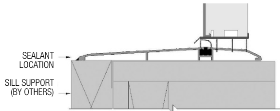
FIG. 17: HANDICAP DOOR SILL
