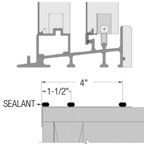
FIG. 11: SLIDING PATIO DOOR SILL
