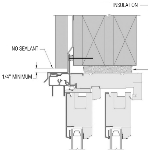
FIG. 25: SLIDING HEAD JAMB
