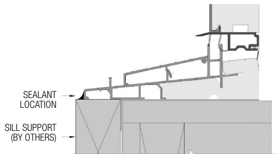
FIG. 16: STANDARD DOOR SILL
