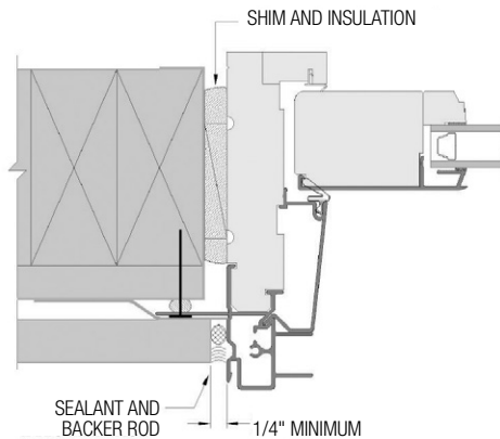
FIG. 24: SIDE JAMB
