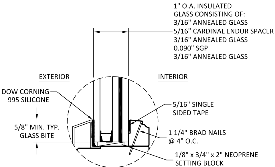
GLAZING DETAIL G2
