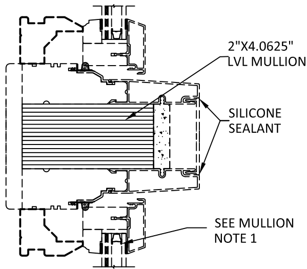
I 3 DUAL CASEMENT OP HORIZONTAL MULLION
