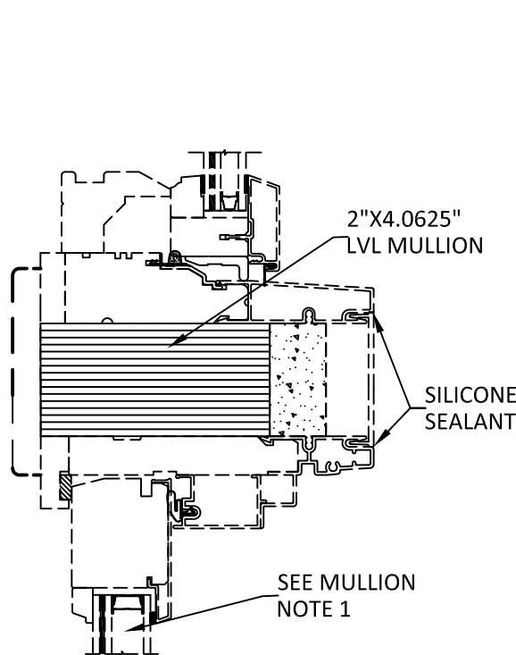
N 3 DH PIC - CASEMENT OP HORIZONTAL MULLION
