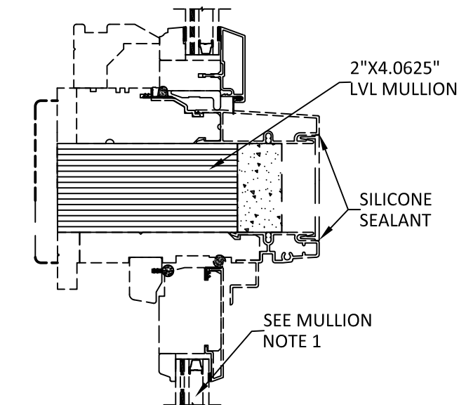
P 3 DH OP - CASEMENT OP HORIZONTAL MULLION
