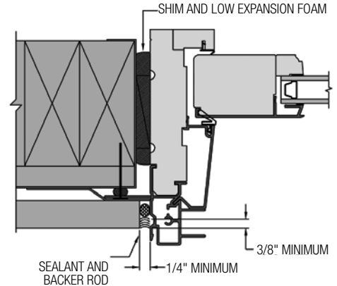
FIG. 23: SIDE JAMB
