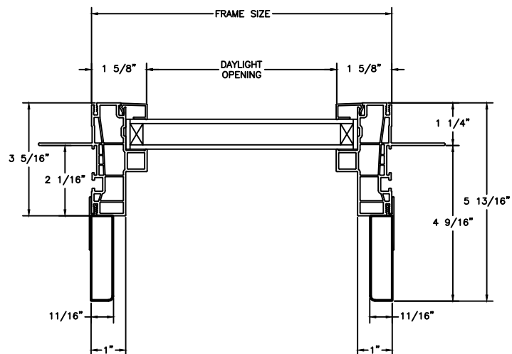
JAMBS
