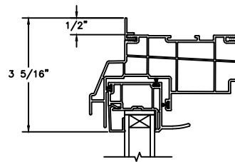
\frac{1}{2}" FLANGE
