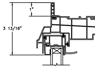
1" FLANGE
