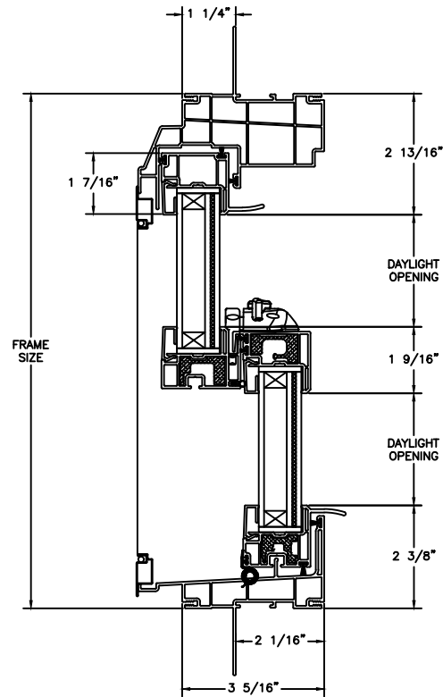
HEAD JAMB & SILL
