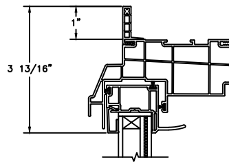
1" FLANGE
