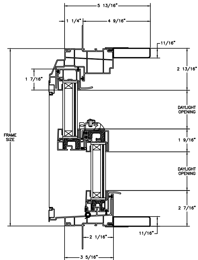
HEAD JAMB & SILL
