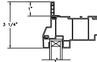
1" FLANGE
