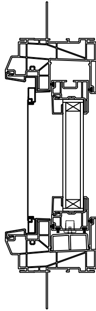
HEAD JAMB & SILL
