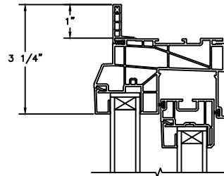
1" FLANGE
