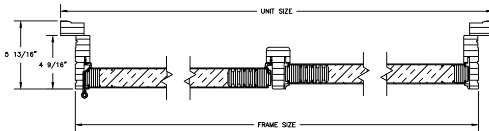
DOUBLE INSWING: 4 9/16 JAMB
