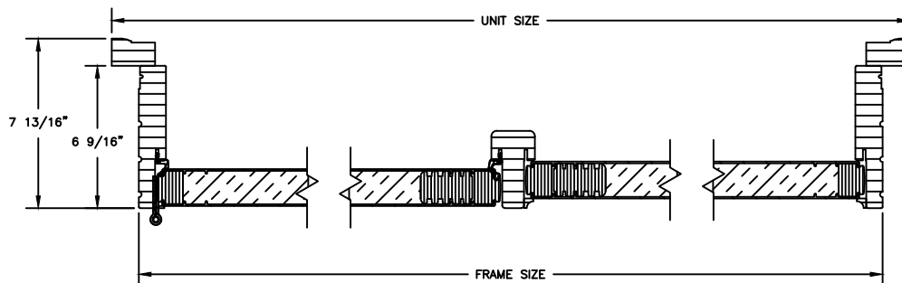
DOUBLE INSWING: 6 9/16 JAMB
