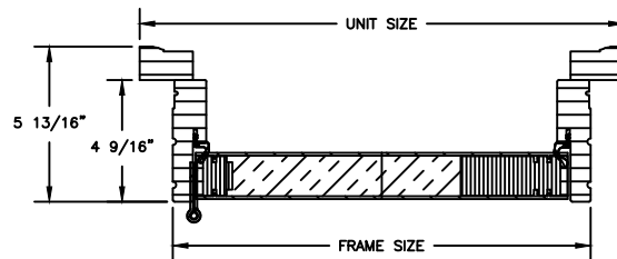
1 PANEL JAMB
