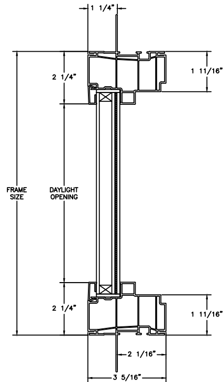
HEAD JAMB & SILL
