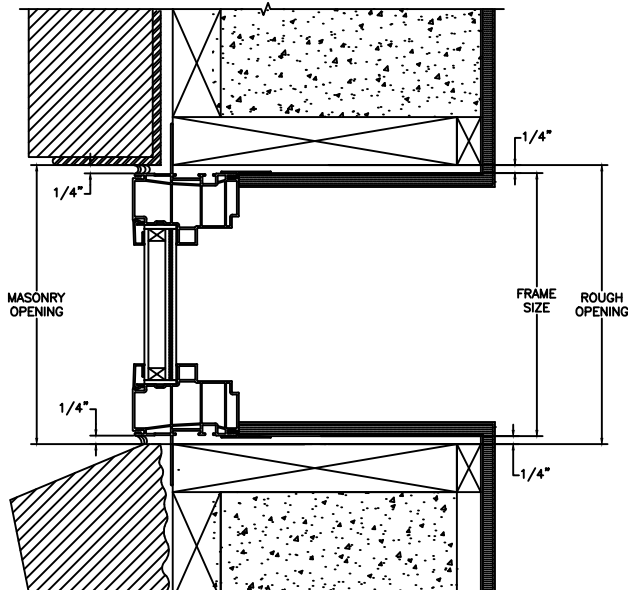
HEAD JAMB & SILL 8\"/>
