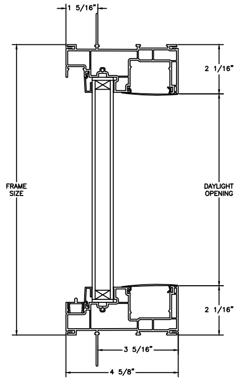
HEAD JAMB & SILL
