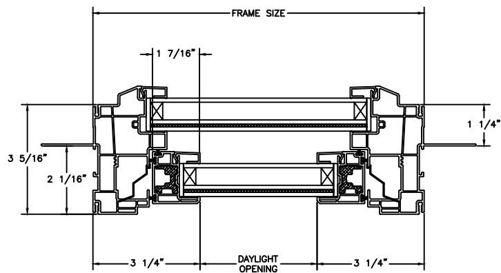
SIDE JAMB
