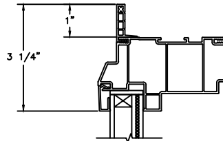
1" FLANGE
