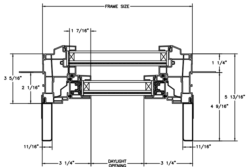
SIDE JAMB
